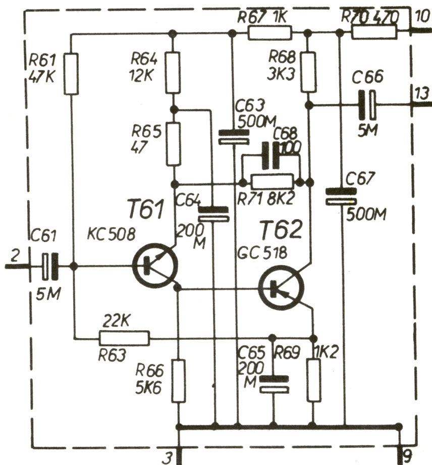
obr. 11. Schéma zapojení mikrofonního zesilovače (3AK 060 44)
