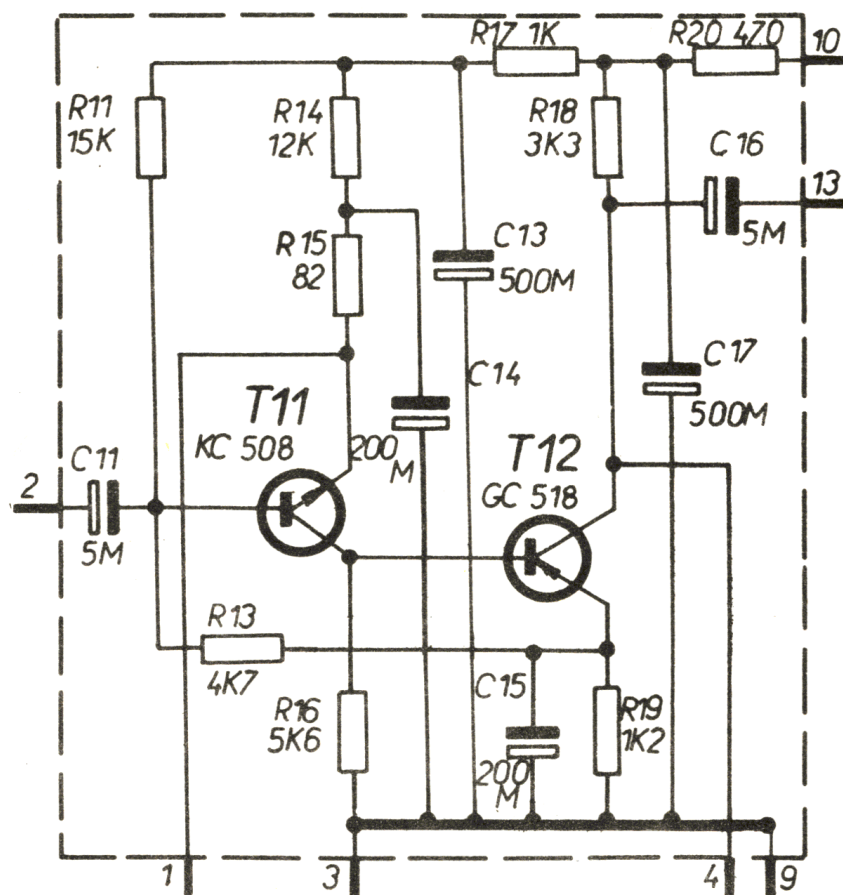
obr. 14. Schéma zapojení směšovacího zesilovače (3AK 060 42)
