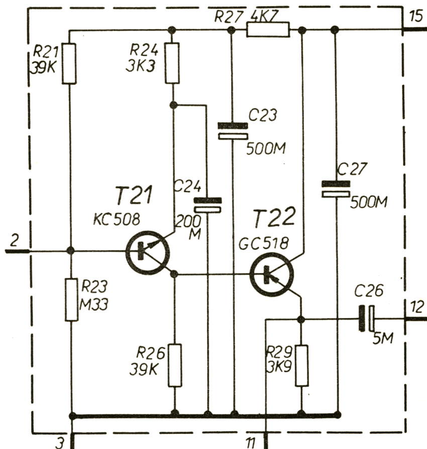
obr. 15. Schéma zapojení korekčního zesilovače (3AK 060 45)
