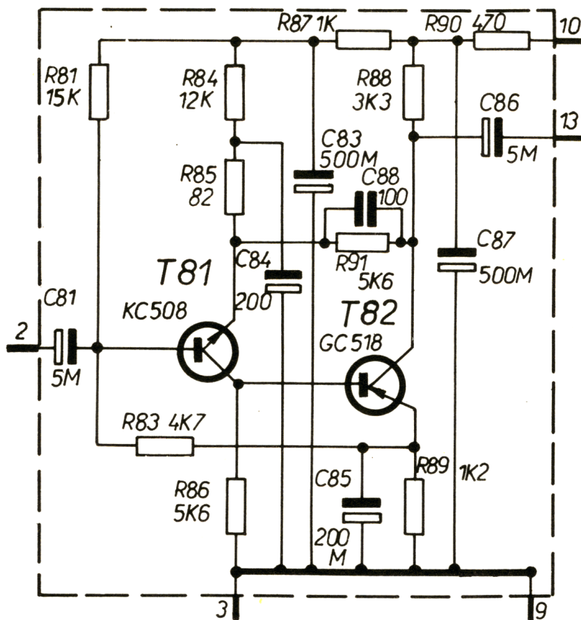
obr. 13. Schéma zapojení směšovacího zesilovače (3AK 060 43)
