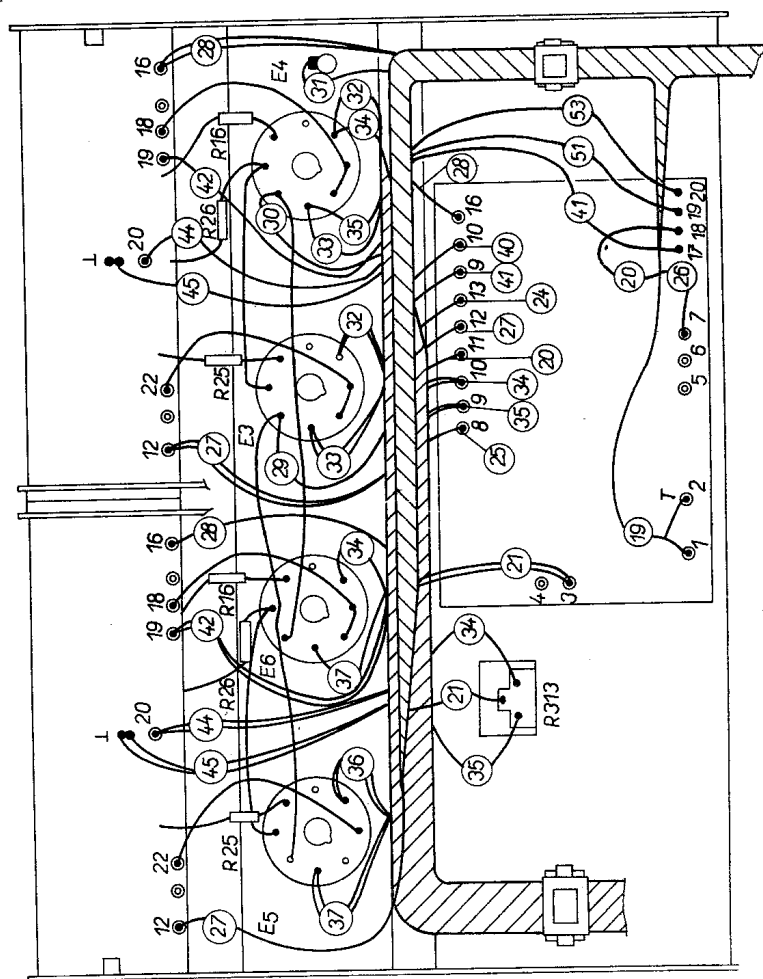
Obr. 20. Zapojení potenciometrů, koncového stupně a napaječe
