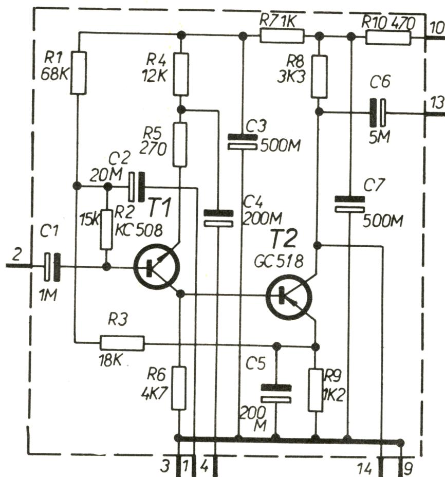
obr. 12. Schéma zapojení univerzálního zesilovače (3AK 060 41)
