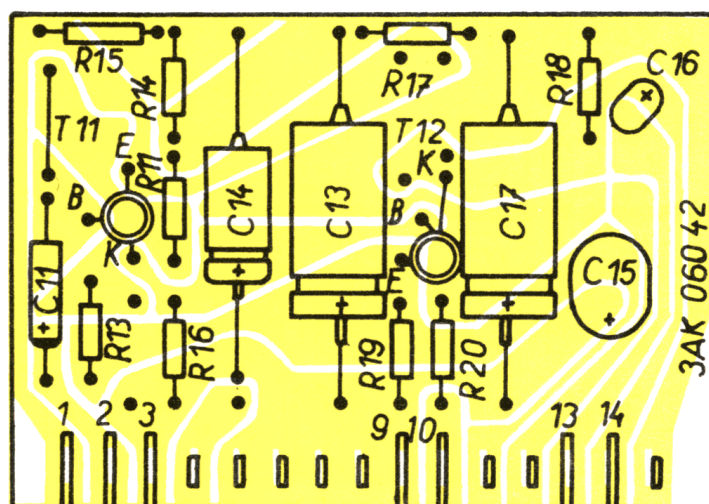
obr. 14a. Zapojení desky směšovacího zesilovače (3AK 060 42)
